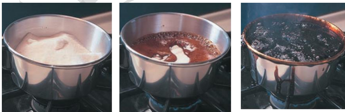
شکل ۲ پ. شکر در اثر گرما تجزیه می‌شود و رنگ آن تغییر می‌کند.
